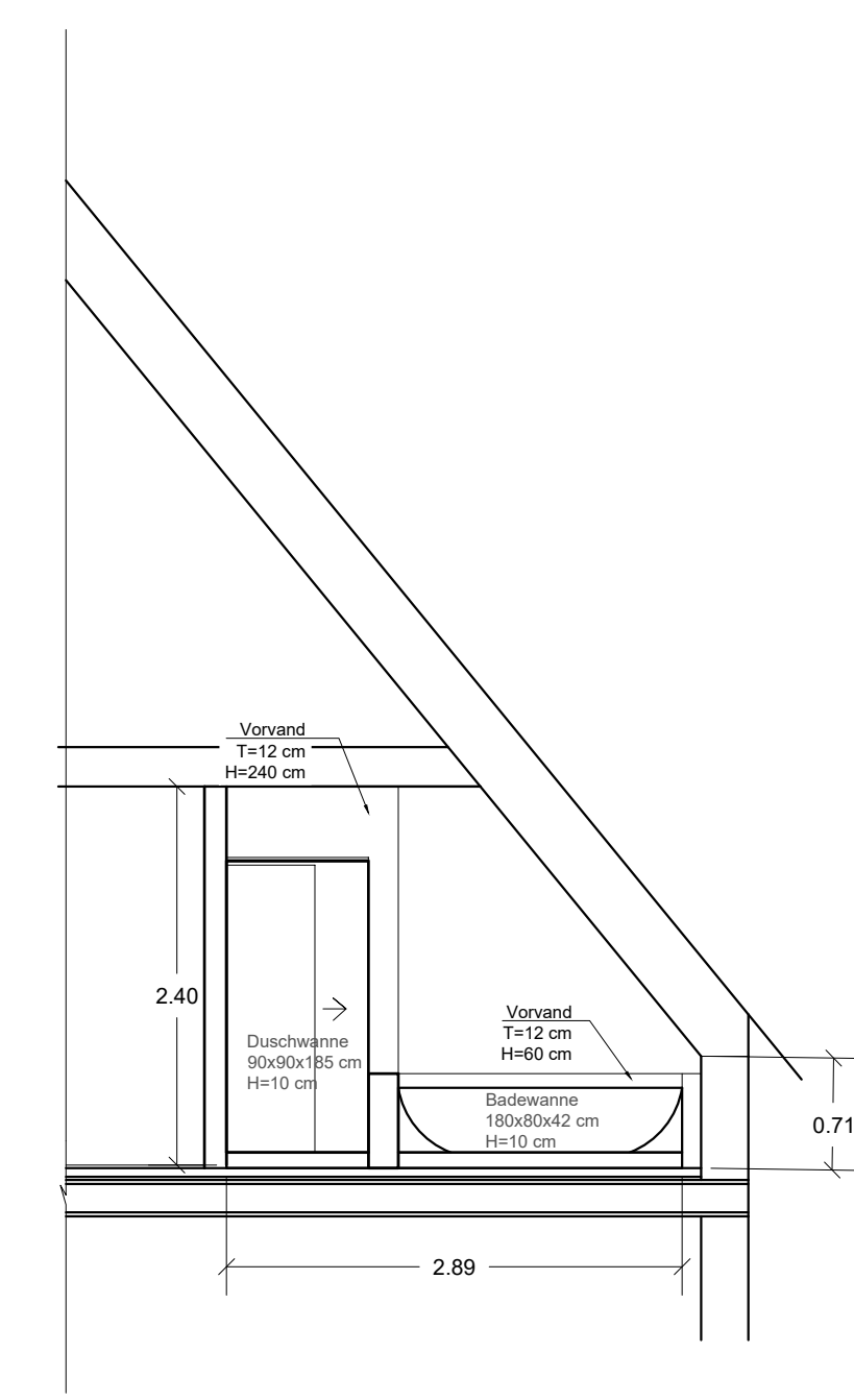
Schnitt R-R M.1:50
