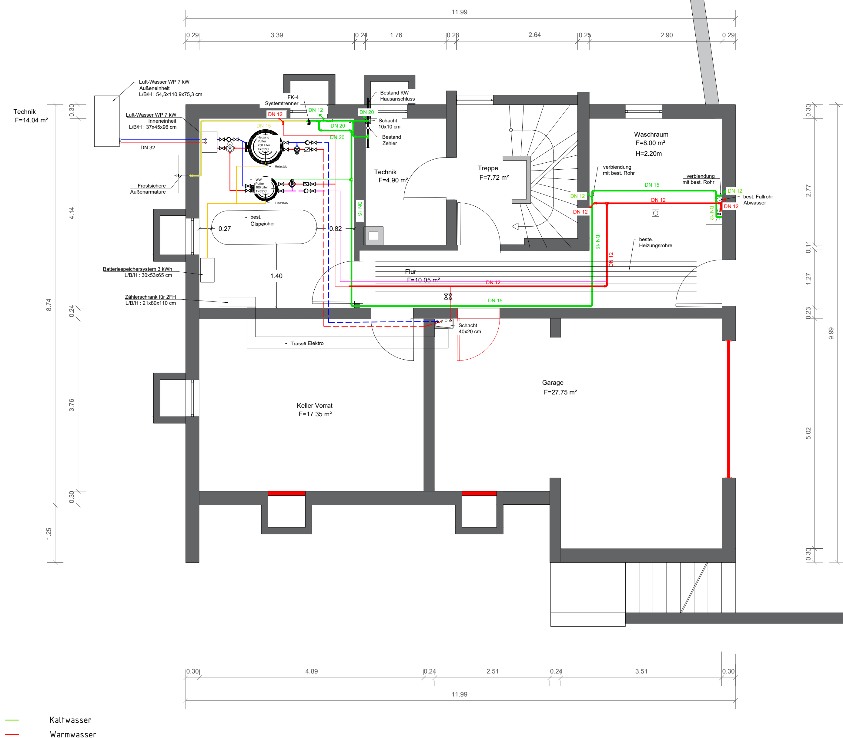
Grundriss EG M.1:50
