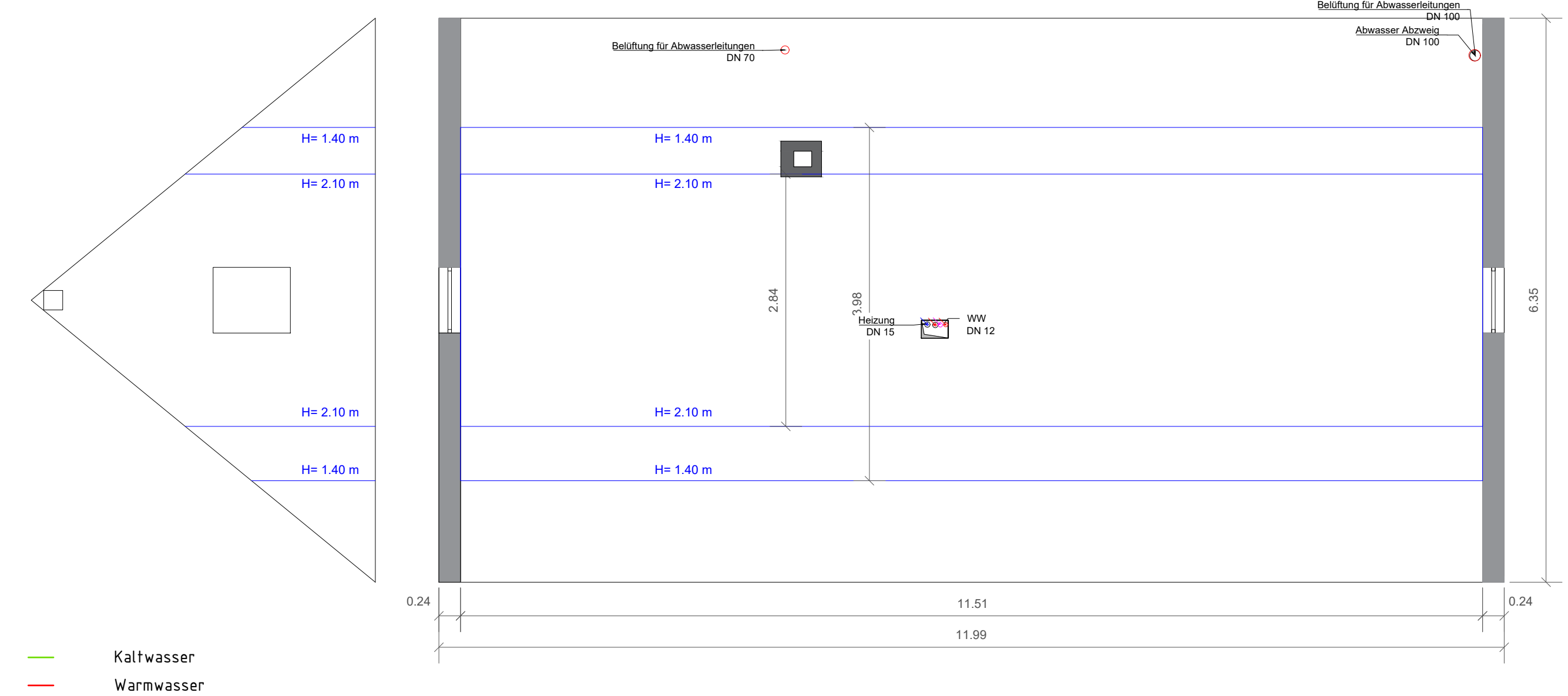
Schnitt R-R M.1:50
